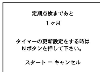
（図2）確認画面
